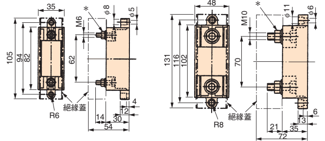
外觀圖 1
