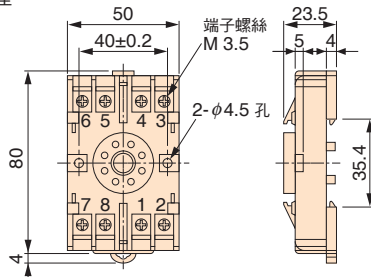
插座
